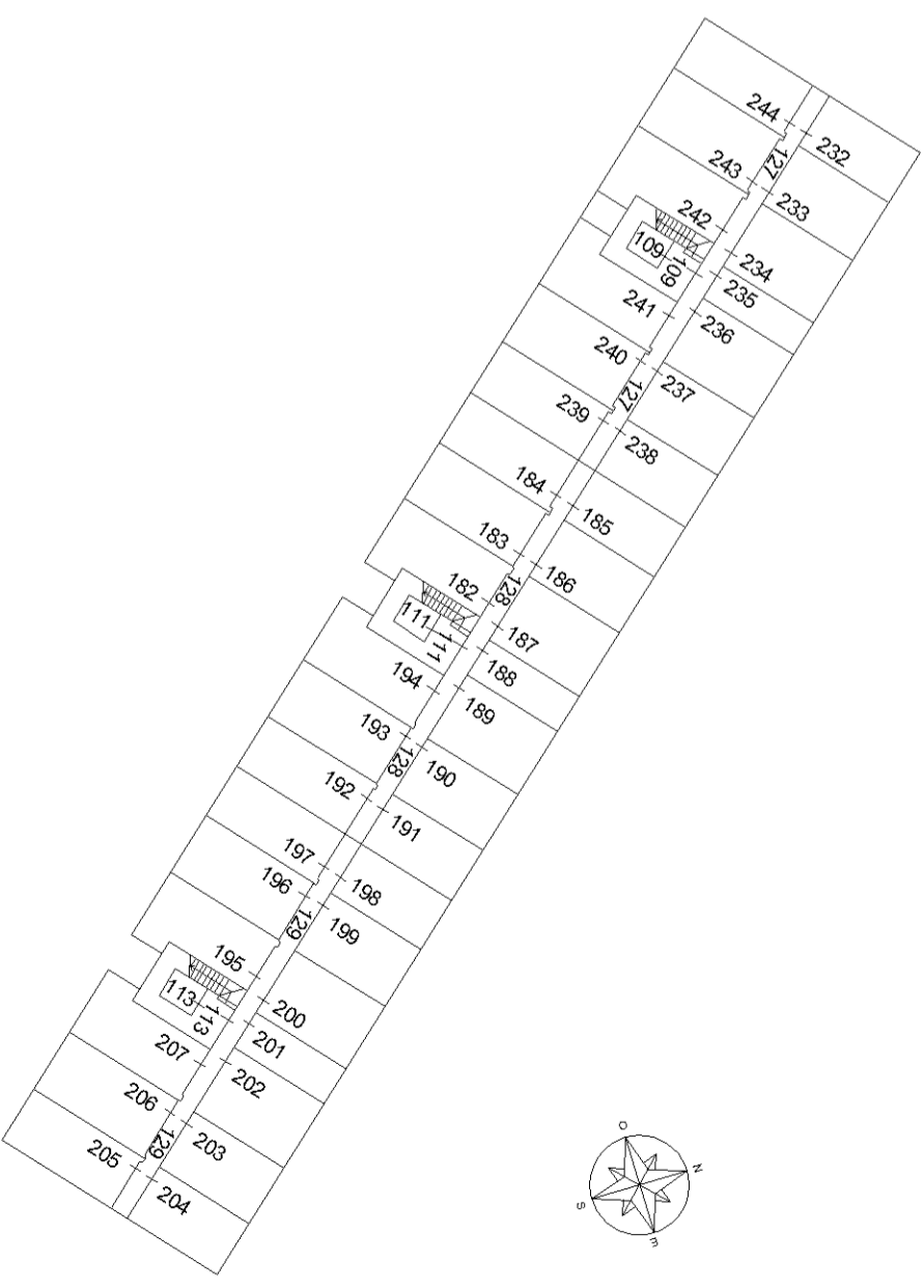
Piano sottostrada 2°
